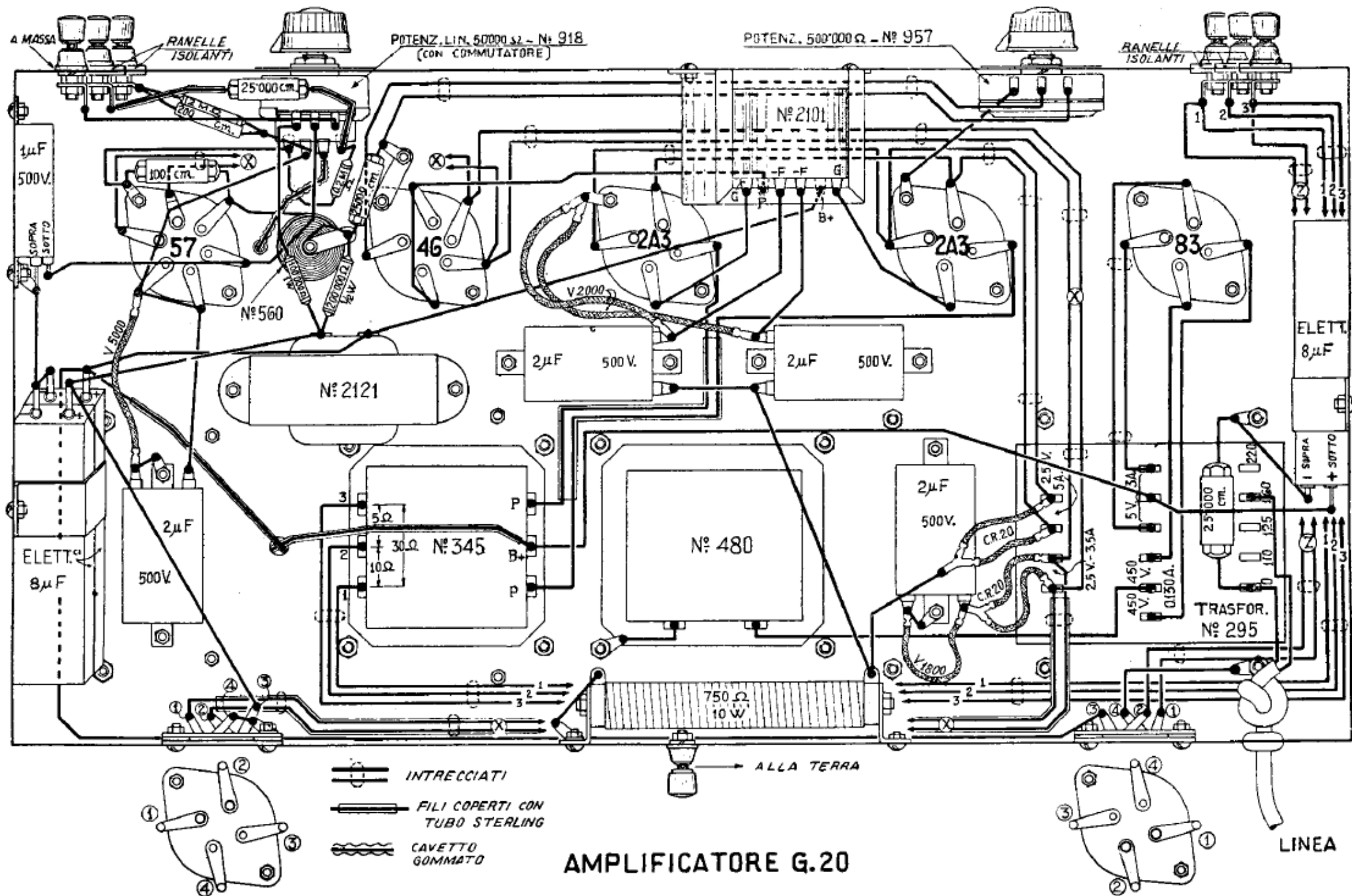
Schema costruttivo dell'amplificatore G-20.
